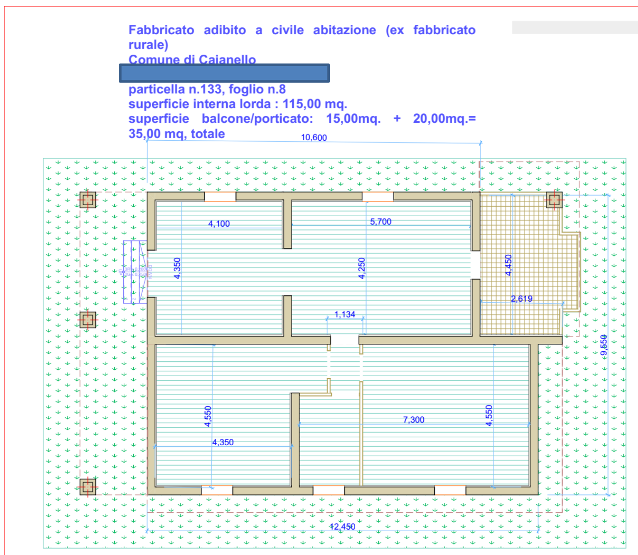
planimetria generale
