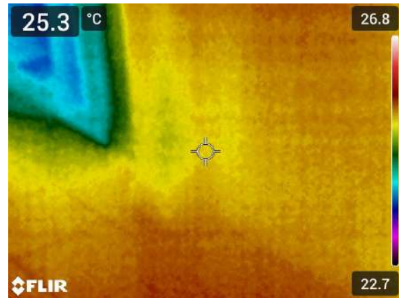
TERMOGRAMMA 2
