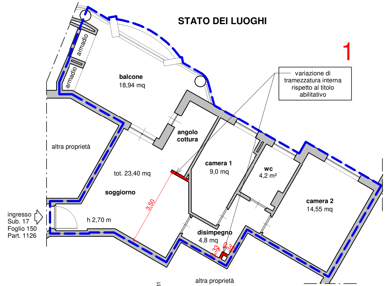
PIANTA Piano Terzo 1 : 100
