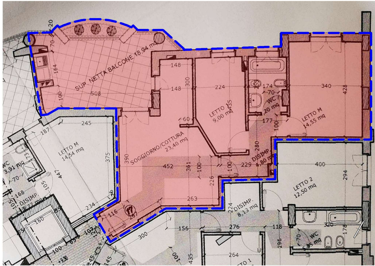
PIANTA Piano Terra 1 : 100
