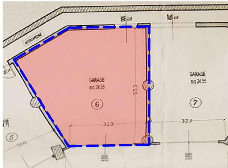
PIANTA Piano Interrato 1 : 100
