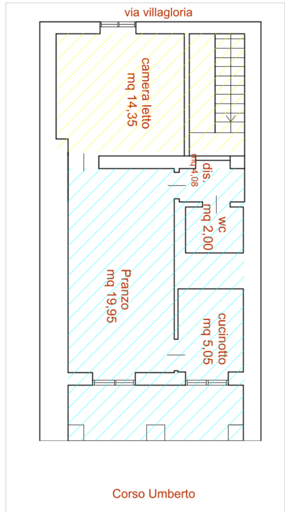
RILIEVO ESEGUITO
