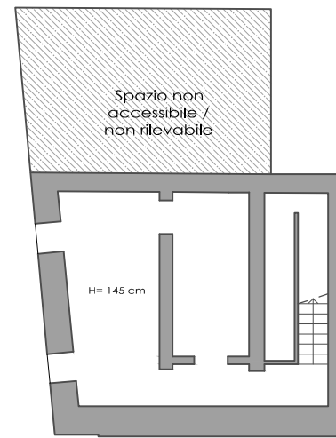
STATO DI FATTO PIANO INTERRATO
