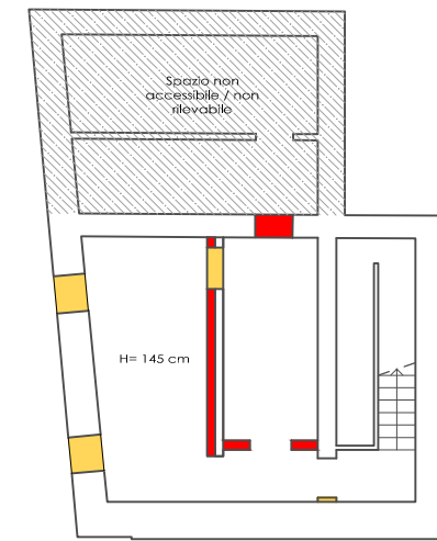
SOVRAPPOSIZIONI PIANO INTERRATO
