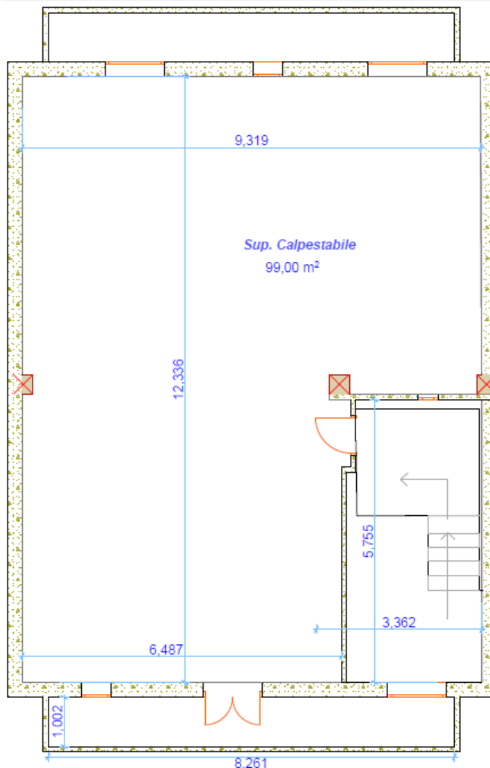
Fig. 30 – planimetria 2° piano
