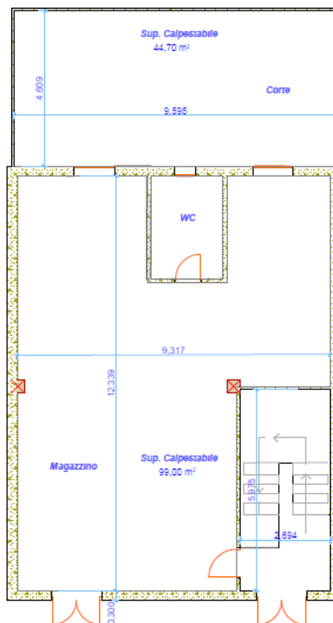
Fig. 9 - planimetria piano terra
