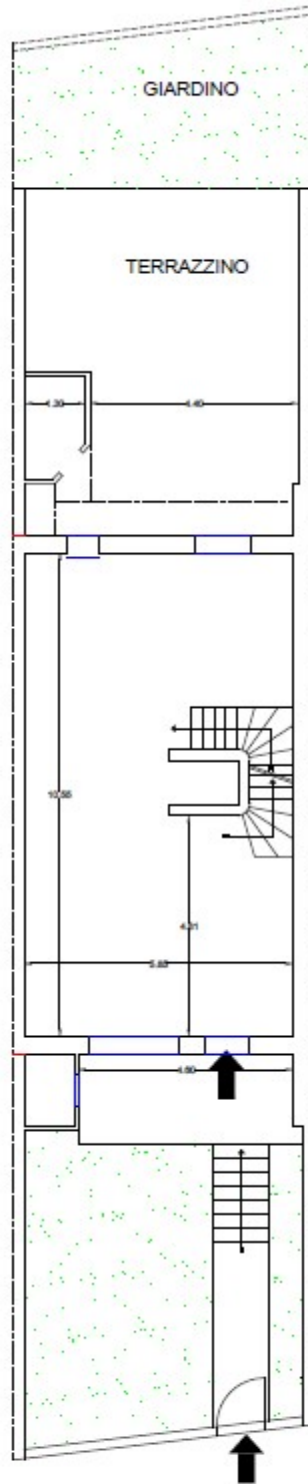
PIANTA PIANO TERRA Fg. 50 part. 2891 sub 6
