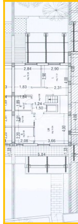
Pianta di progetto P.1°
