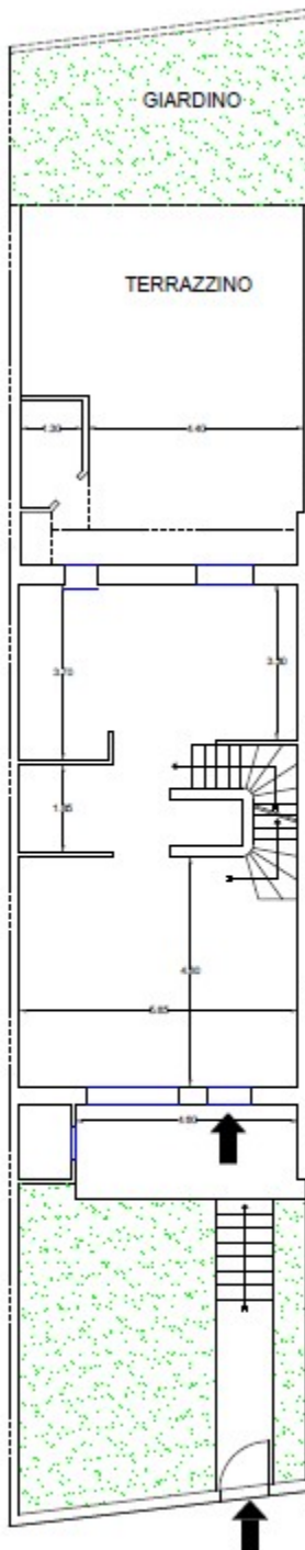
PIANTA PIANO TERRA Fg. 50 pat. 2891 sub 4
