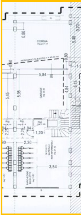
Pianta di progetto S1
