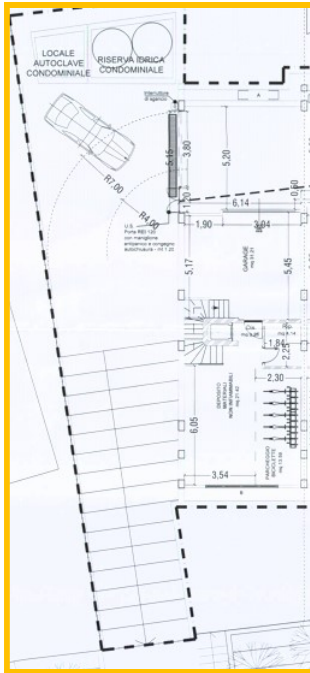
Pianta di progetto S1
