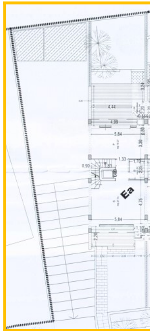
Pianta di progetto P.T.
