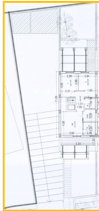
Pianta di progetto P.1°
