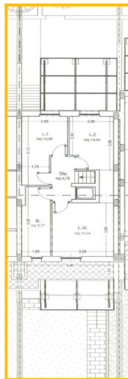
Pianta di progetto P.1'
