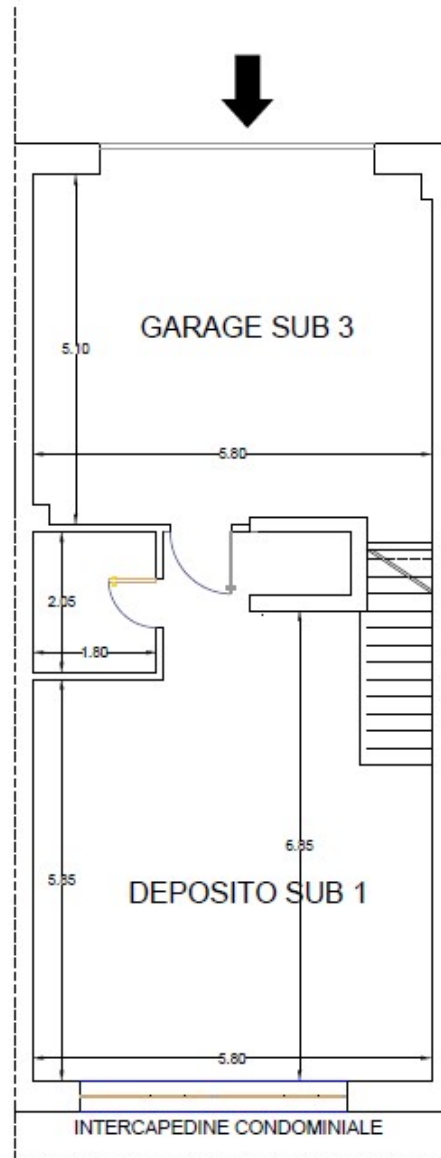
PIANTA PIANO INTERRATO Fg. 50 pat. 2816 sub 1-3
