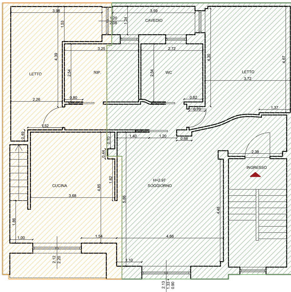
PIANO RIALZATO - scala 1:100
