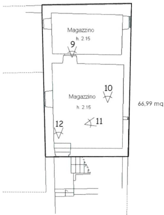
PIANO PRIMO
