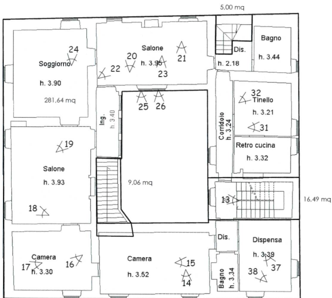
PIANO SECONDO
