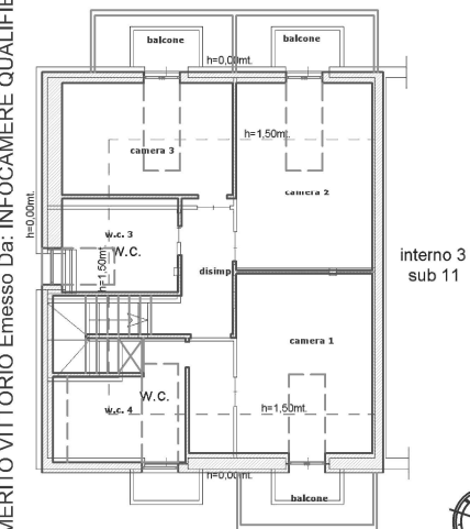
PIANTA PIANO TERZO Hmedia=2,00MT.
