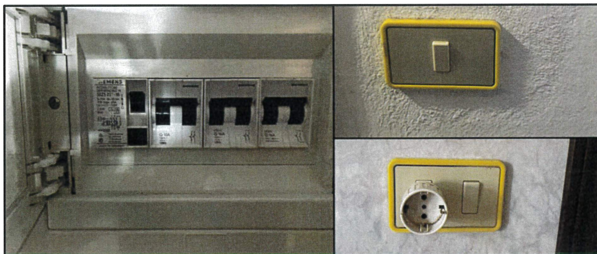
Impianto elettrico: quadro all'interno dell'immobile e dettagli dell'impianto stesso.
