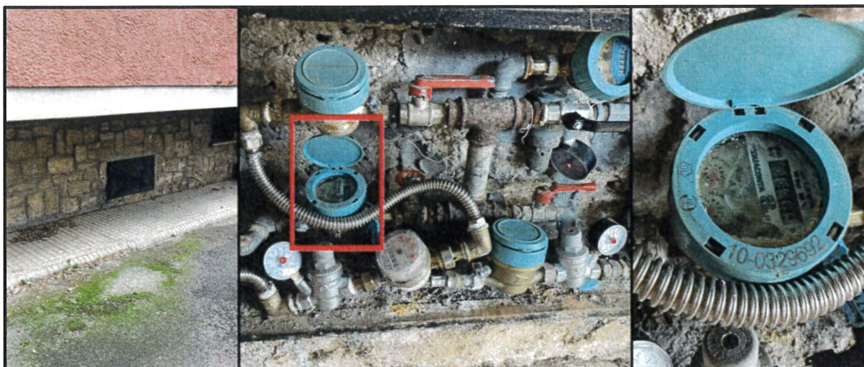
Impianto idrico: punto di fornitura e alloggiamento contatori
