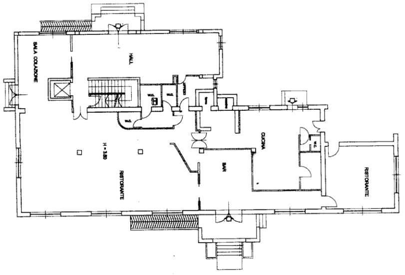
PIANTA PIANO RALZATO
