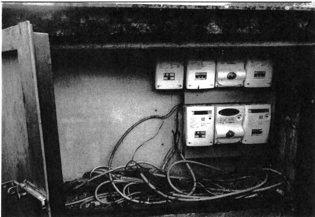
Foto 27 – vano dei contatori dell'energia elettrica posto nella parte esterna del muro di confine sul lato sinistro dell'ingresso dal parcheggio pubblico
