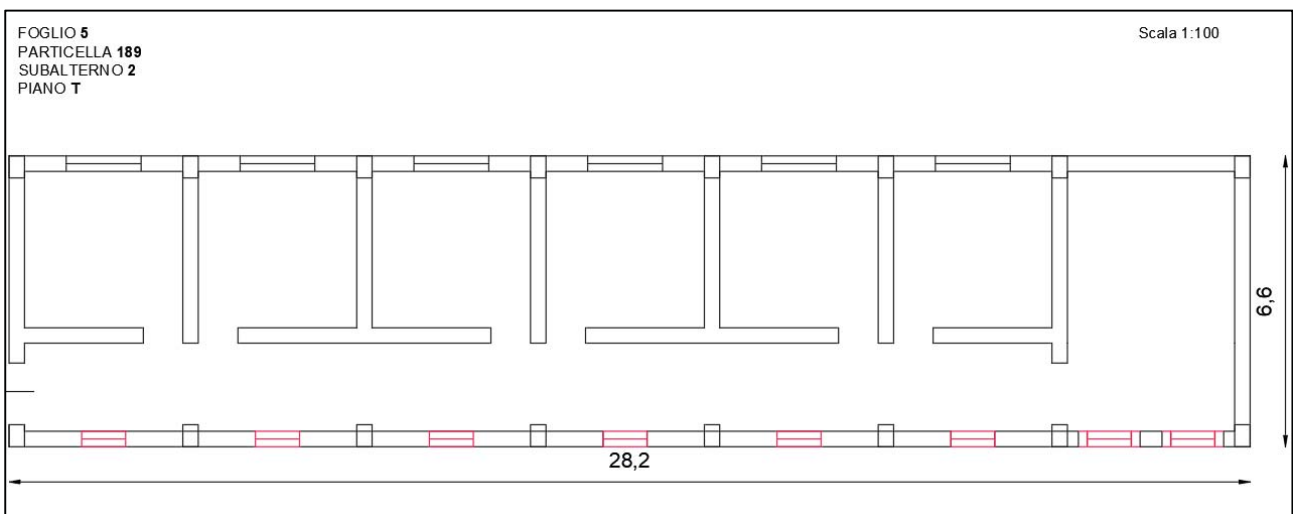
Fig. 15 – Planimetria incongruenze catastali Sub 2- Piano0
