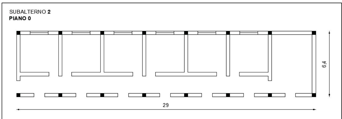
Fig. 8 – Planimetria dell'immobile sub 2
