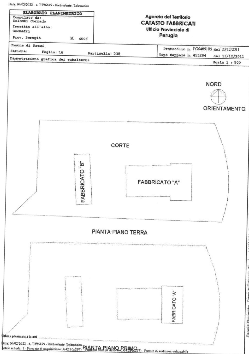
Elaborato planimetrico foglio 16 particella 238
