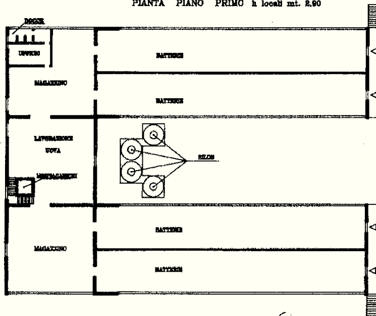
PIANTA PIANO PRIMO h locali mt. 2,80
