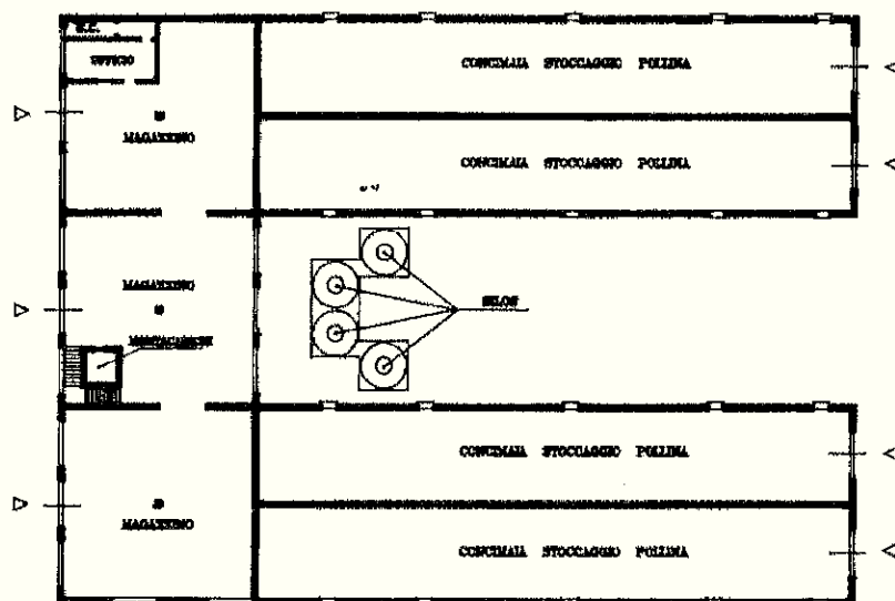
PIANTA PIANO TERRA h locali mt. 2,70
