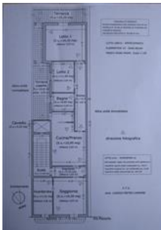
Pianta dell'immobile esistente
