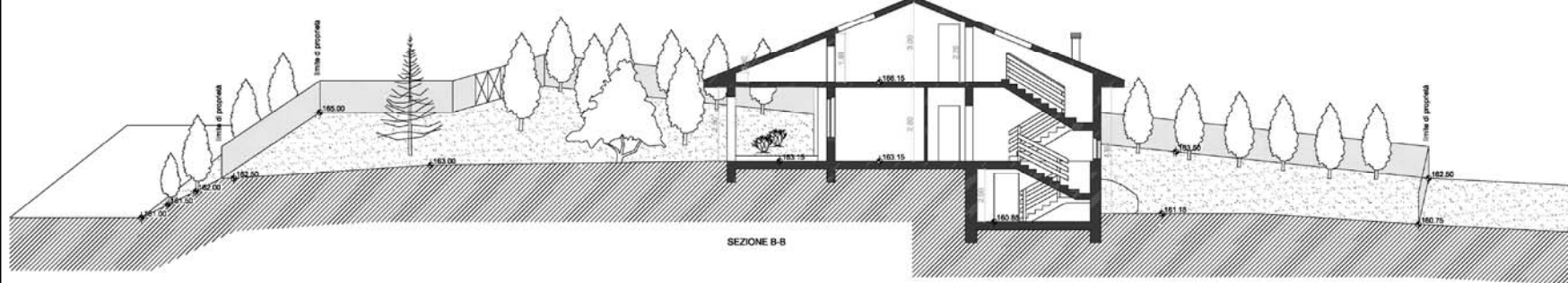
sezione B-B
