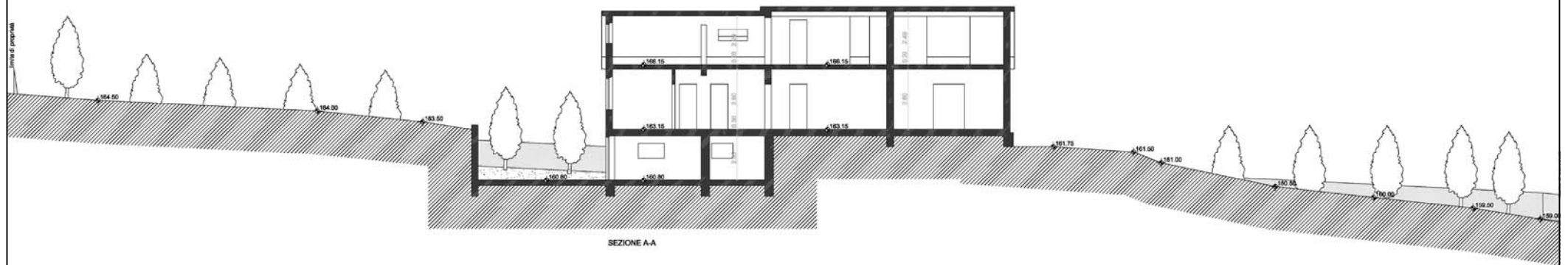
sezione A-A
