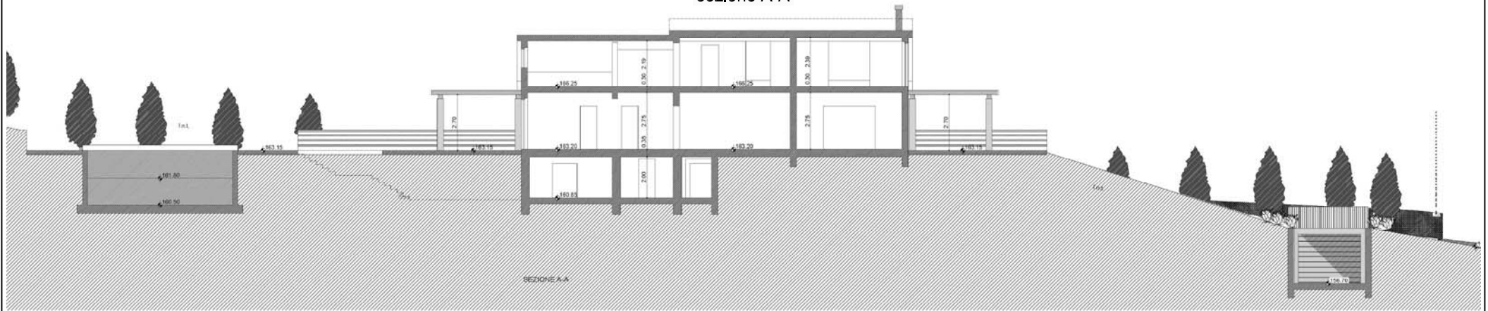
sezione A-A
