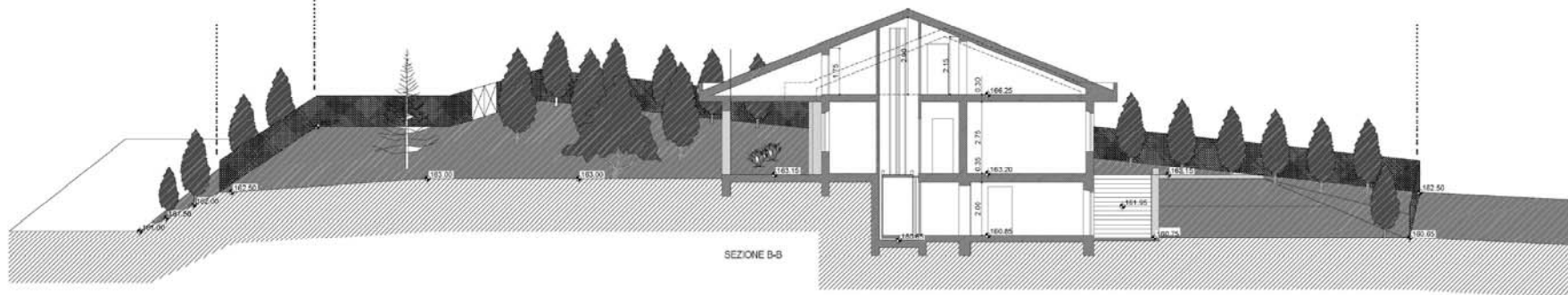
sezione B-B
