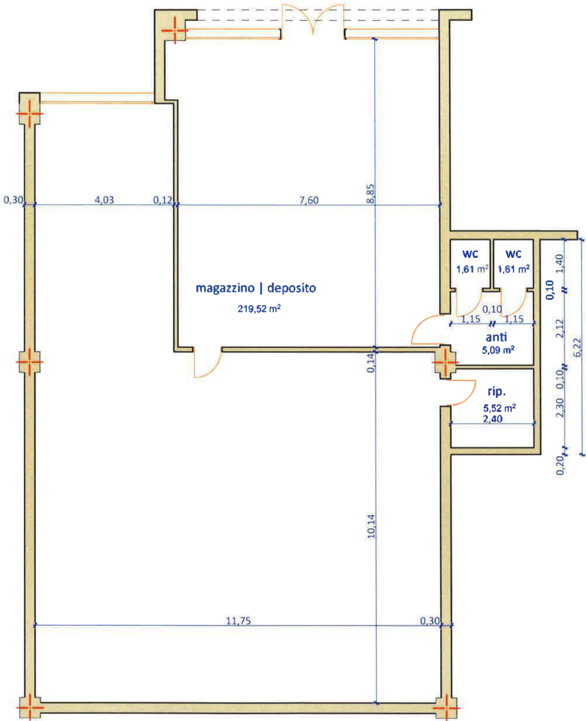
lotto 002 _magazzino | deposito — piano terra _rilievo —sup. lorda mq 245,63 scala 1:100
