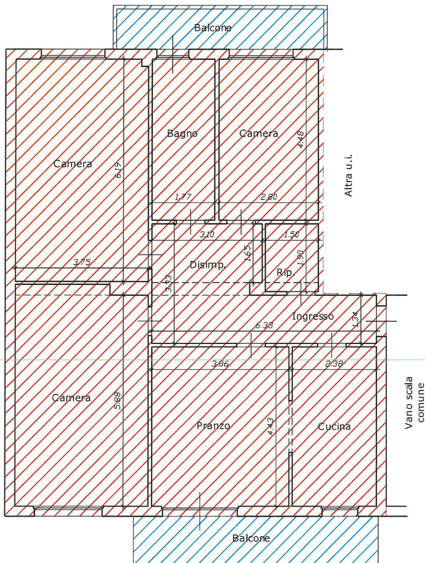
PIANO PRIMO H. 3,05 mt.
