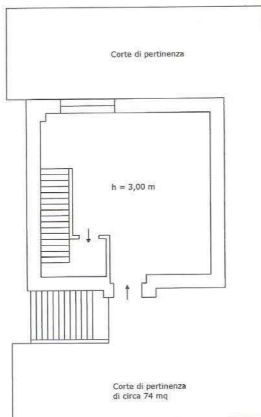
Planimetria Piano Terra Scala 1:100
