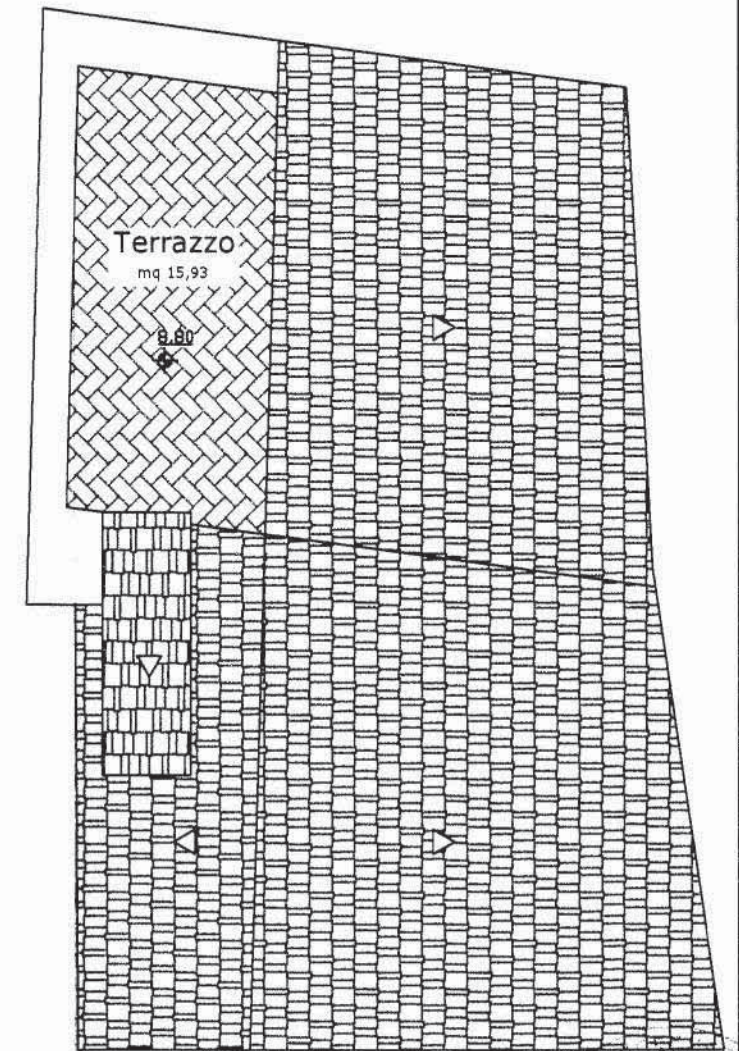
Piano copertura
