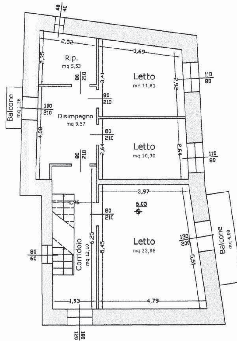
Piano primo
