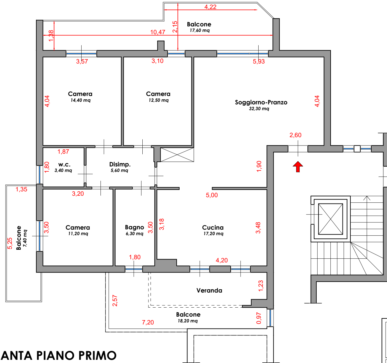
PIANTA PIANO TERRA H= 2,70 m
