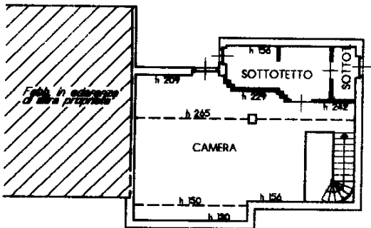
SOTTOTETTO Hmedia= 240
