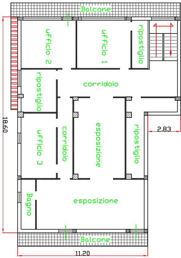
PIANO SECONDO SOTTOTETTO Scala 1:200 [H=2.39] [STATO ATTUALE]
