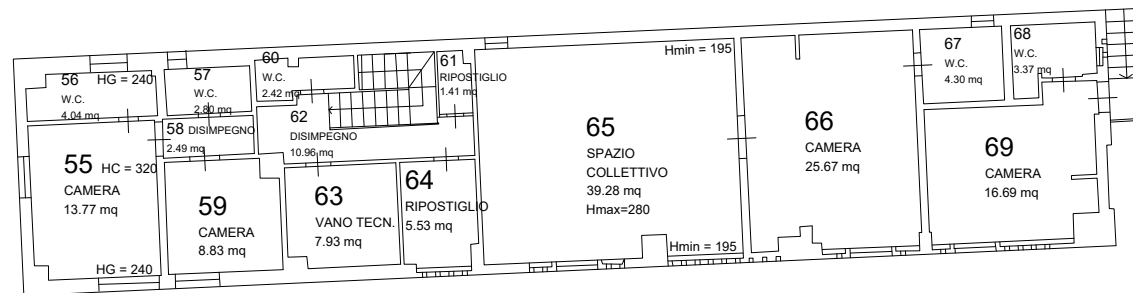
PIANO PRIMO Pianta fabbricato accoglienza agrituristica
