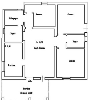
Pianta da rilievo scala 1:100
