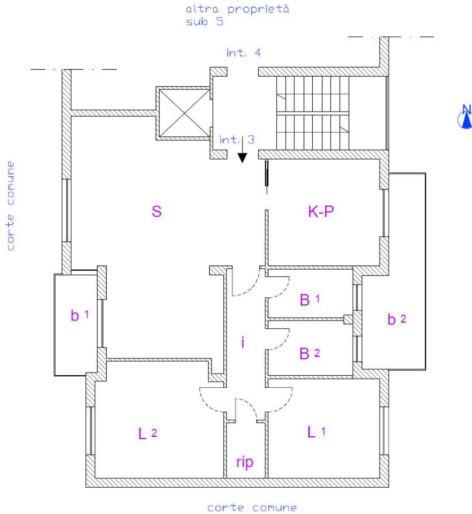
Planimetria dello stato di fatto – sub 4 - appartamento
