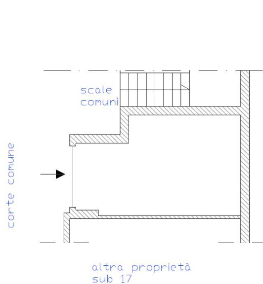
Planimetria dello stato di fatto – sub 18 – box auto
