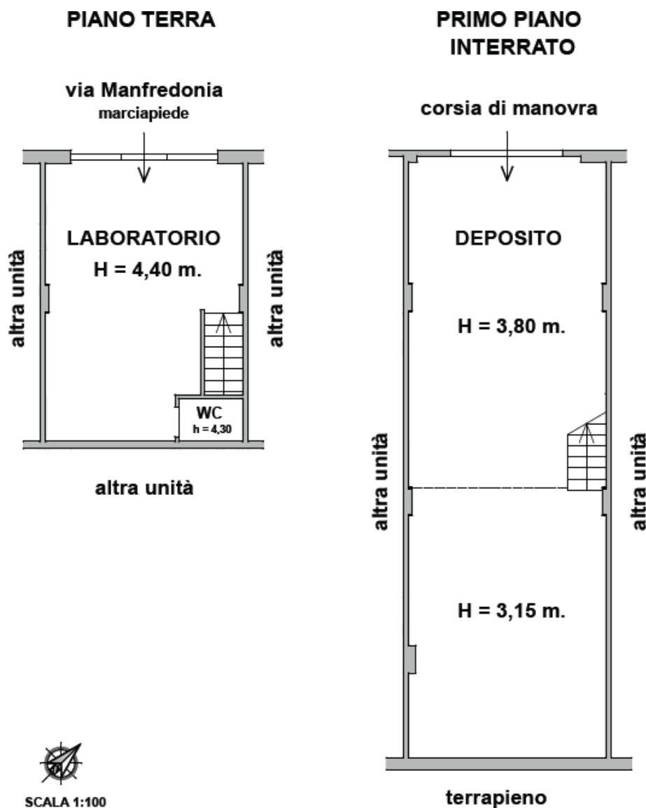
Fig. 2 - LOTTO 1 - Planimetria laboratorio artigianale foglio 52 - part. 604 - sub. 13
