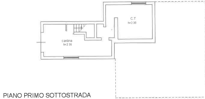
PIANO PRIMO SOTTOSTRADA
