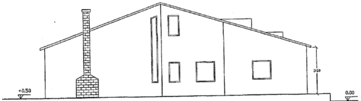
PROSPETTO NORD
