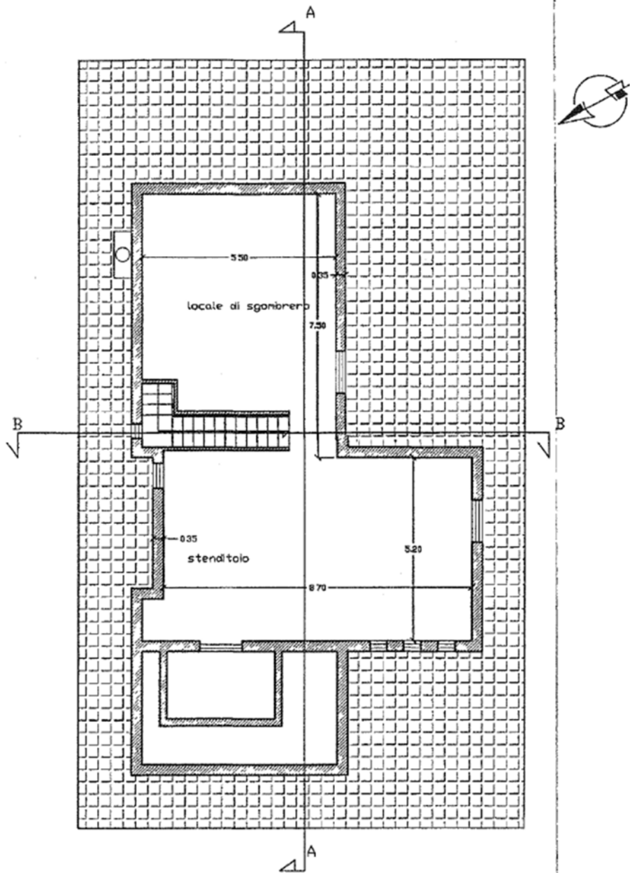
PIANTA SOTTOTETTO
