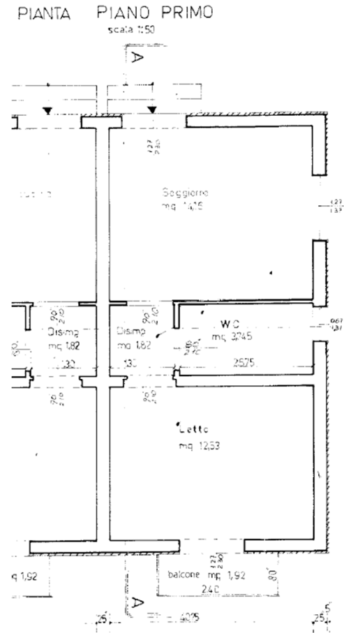
Planimetria stato di progetto
