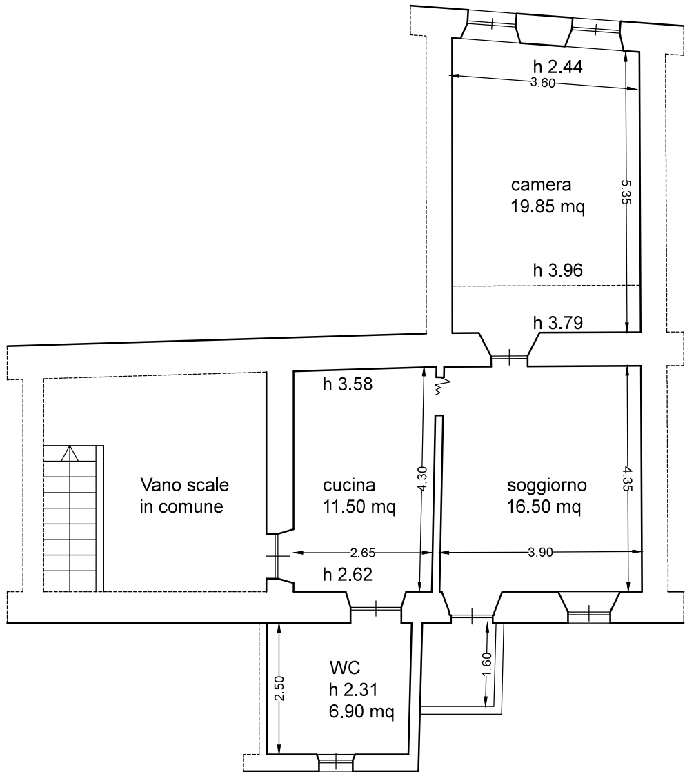
Planimetria appartamento piano secondo stato rilevato
