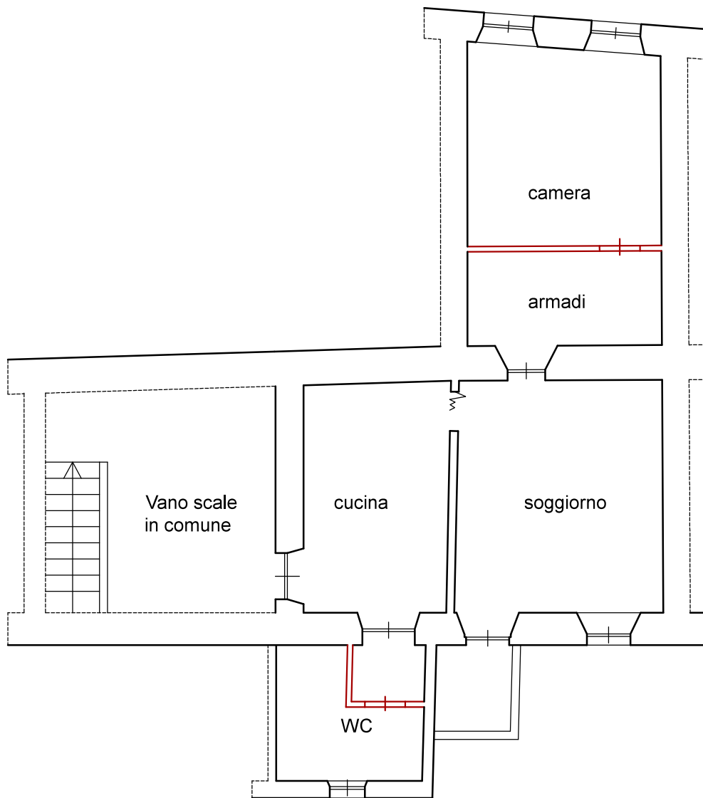
Planimetria sovrapposto
