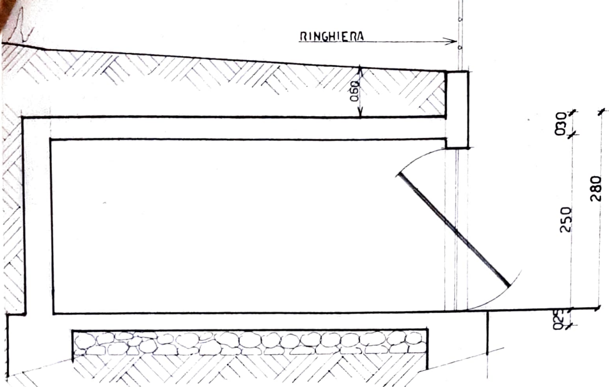
PARTICOLARE SEZIONE DEL SINGOLO BOX SCALA 1:50
