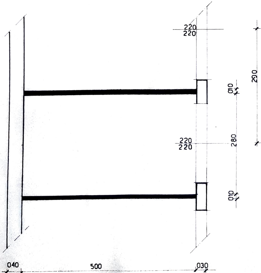
PARTICOLARE PIANTA DEL SINGOLO BOX SCALA 1:50
