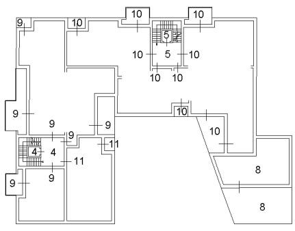
PIANO PRIMO H. 2.70 mt
