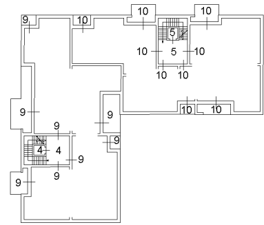
PIANO SECONDO H. 2.70 mt
