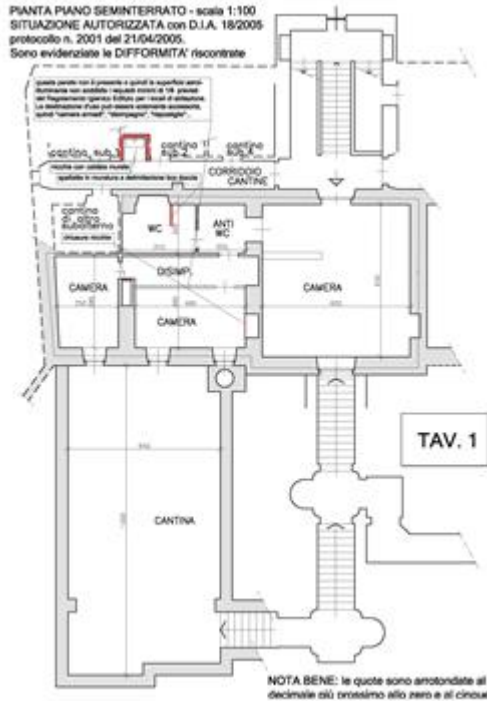
planimetria con l'autorizzato e evidenziazione delle difformità riscontrate
