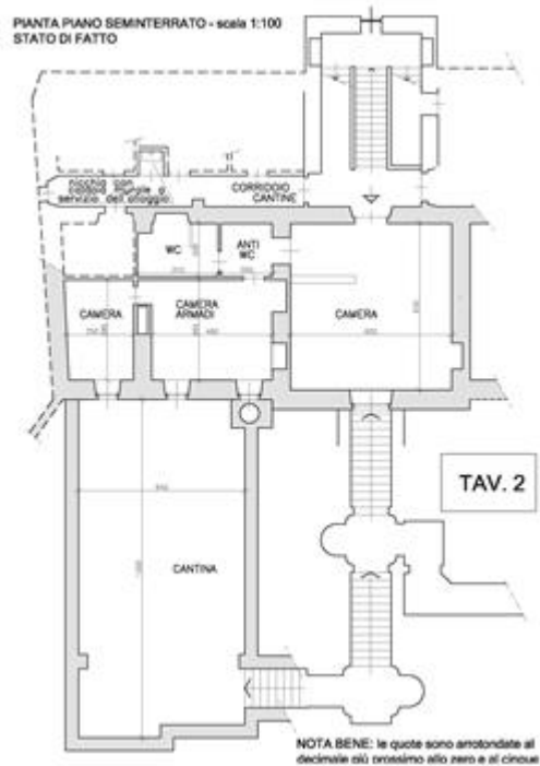
planimetria dello stato di fatto
