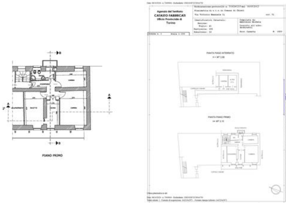
Planimetria catastale in cui è rappresentata anche la cantina
