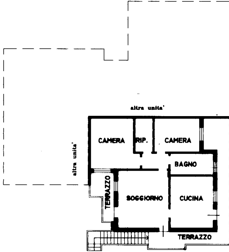
PIANTA PIANO PRIMO h=2.70m
