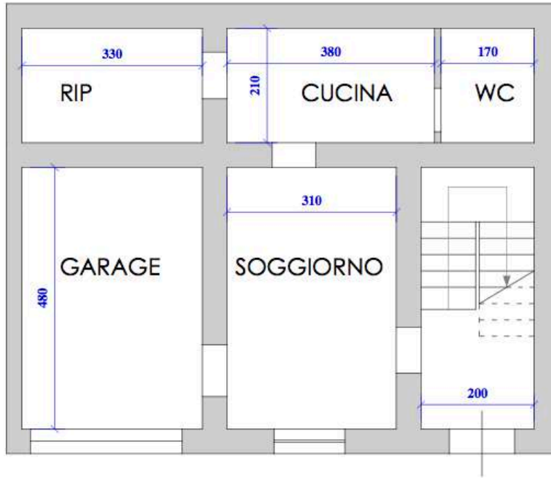
PLANIMETRIA DEL PIANO TERRA
