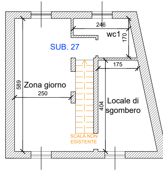
PIANO PRIMO scala 1:100
