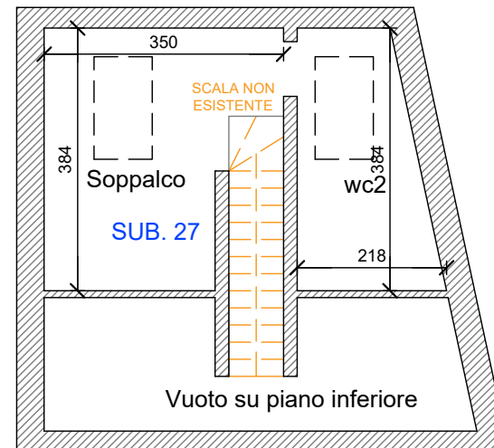
PIANO SOTTOTETTO scala 1:100
