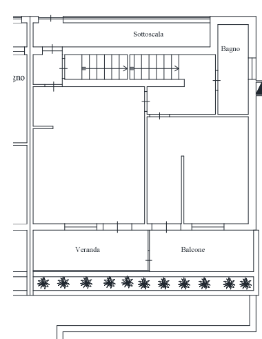
Rilievo piano seminterrato da demolire
