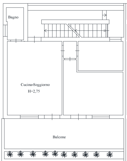
Rilievo piano secondo
