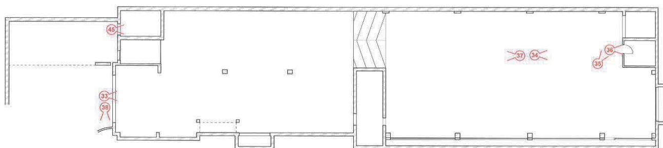
PIANTA PIANO PRIMO Scala 1:200
