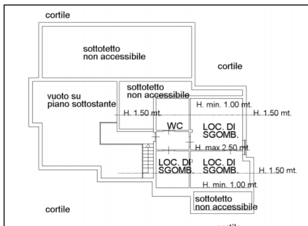
Planimetria piano terreno estratta dall'elaborato catastale
