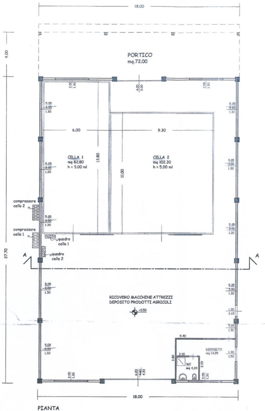
Planimetria Piano terra capannone agricolo – STATO ATTUALE
