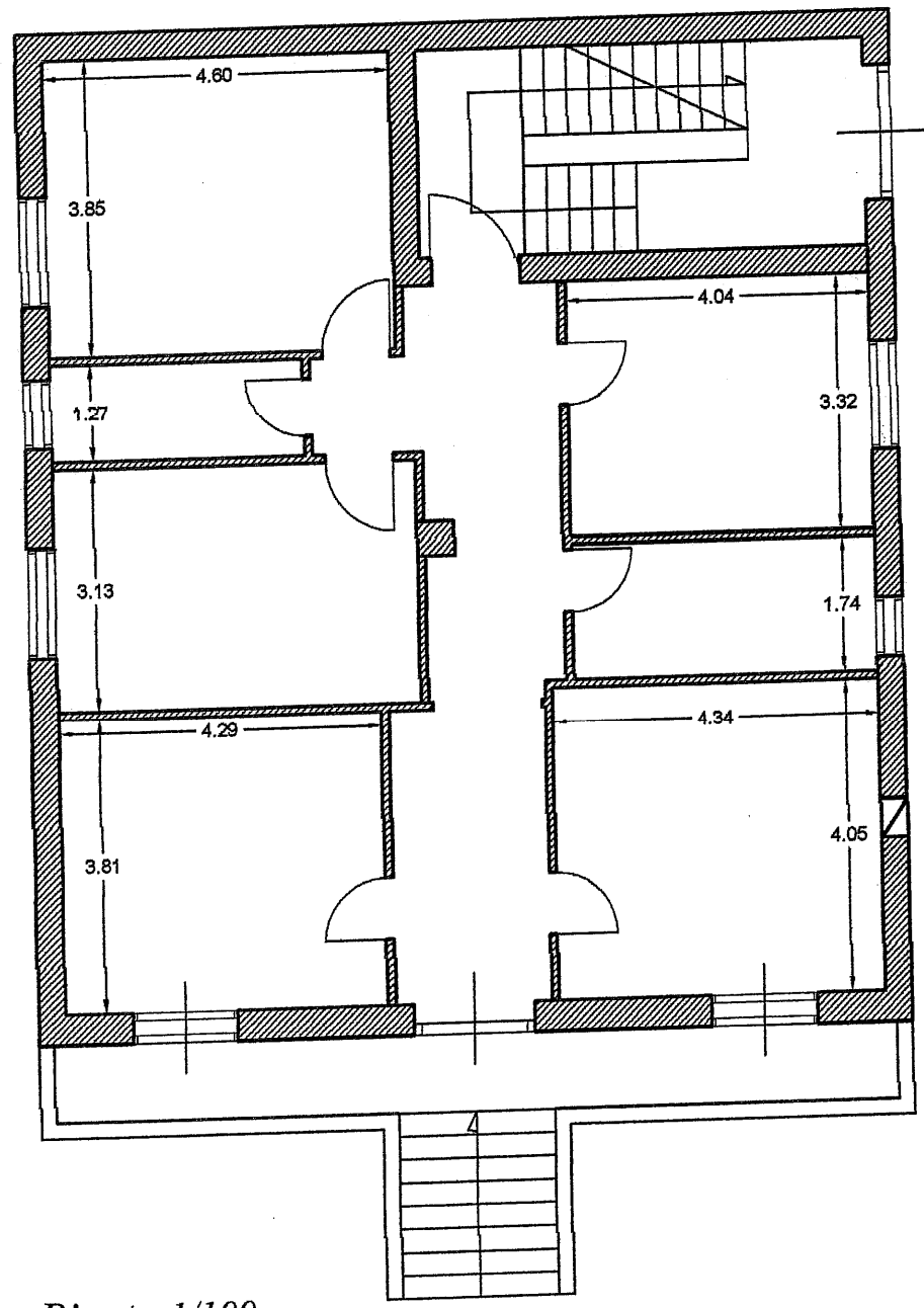
Pianta 1/100
