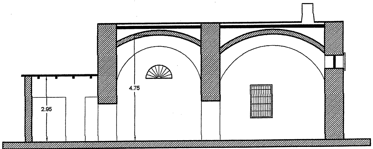
Sez A-A' 1/100
