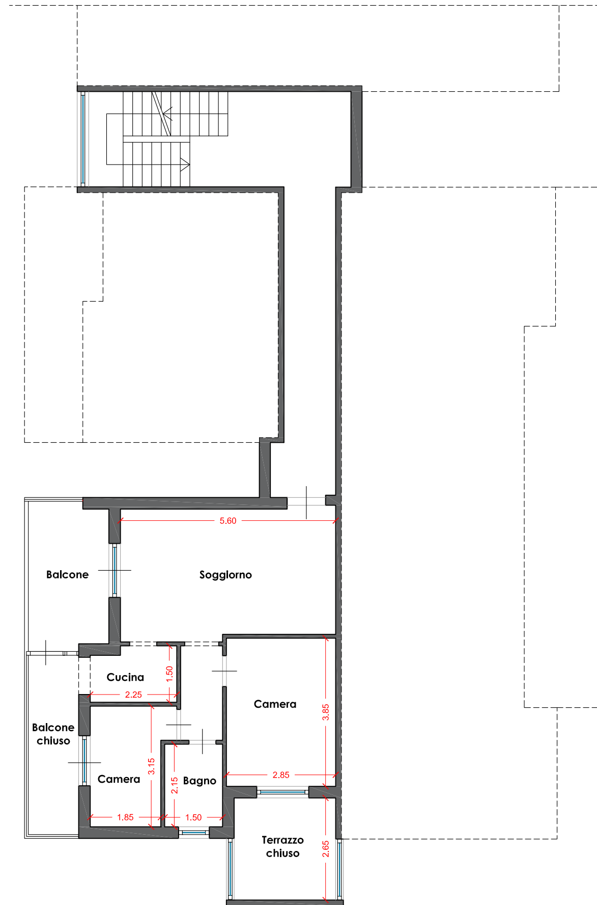
PIANTA PIANO PRIMO H= 2.80m
